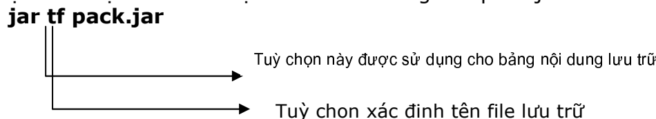
Hình 10.1 lệnh jar
