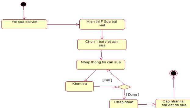
Hình 2.10. Biểu đồ hoạt động sửa bài viết
