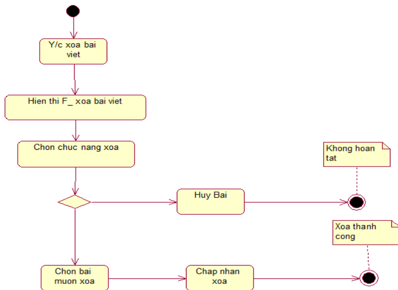
Hình 2.11. Biểu đồ hoạt động xóa bài viết
