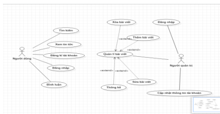
Hình 2.1. Biểu đồ usecase
