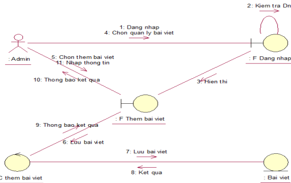
Hình 2.8. Biểu đồ cộng tác cho ca sử dụng thêm bài viết
