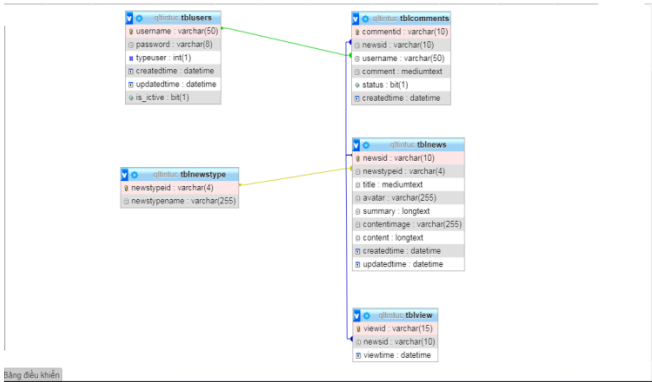
Hình 3. 1. Quan hệ giữa các bảng
