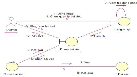
Hình 2.6. Biểu đồ cộng tác cho ca sử dụng xóa bài viết
