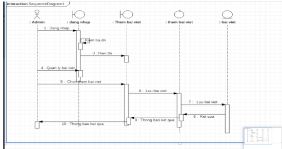
Hình 2.5. Biểu đồ trình tự cho ca sử dụng thêm bài viết
