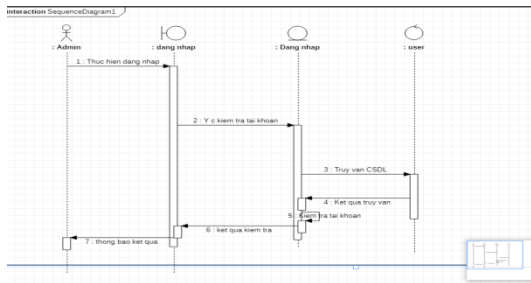
Hình 2.3. Biểu đồ trình tự cho ca sử dụng đăng nhập
