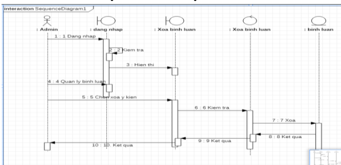
Hình 2.4. Biểu đồ trình tự cho ca sử dụng xóa bình luận
