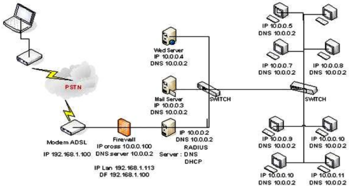
Hình 6.5 - Mô hình Firewall cơ bản thường được sử dụng
