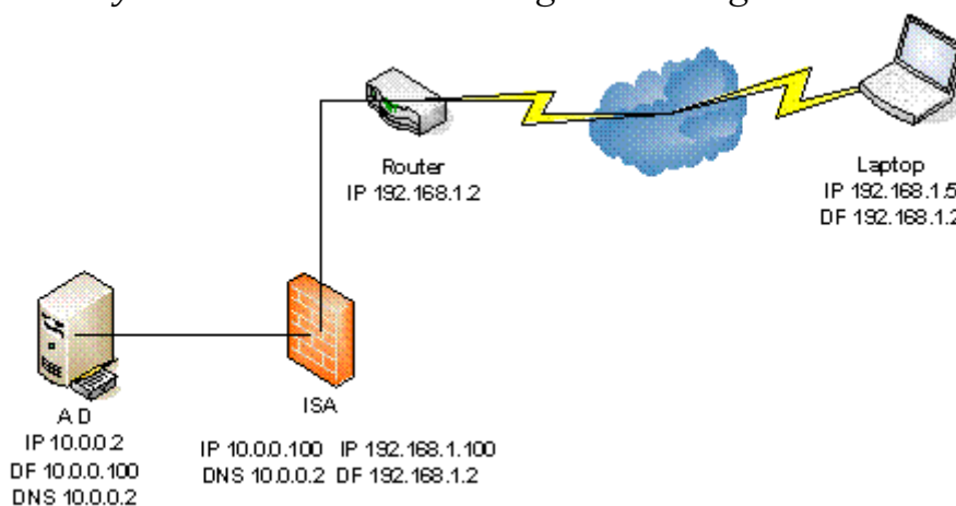
Hình 8.26 - Mô hình VPN Client to Site dùng giao thức L2TP/IPSEC
