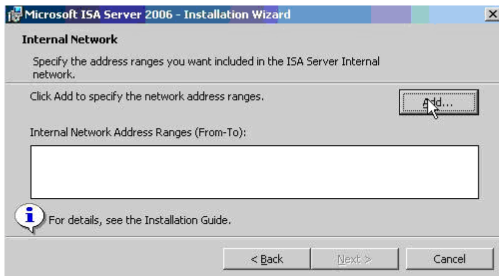
Hình 7.1 - Định nghĩa vùng Internal Network
