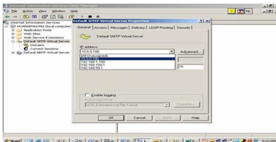
Hình 9.16 – Thiết lập đối với Default SMTP Virtual Server Properties
