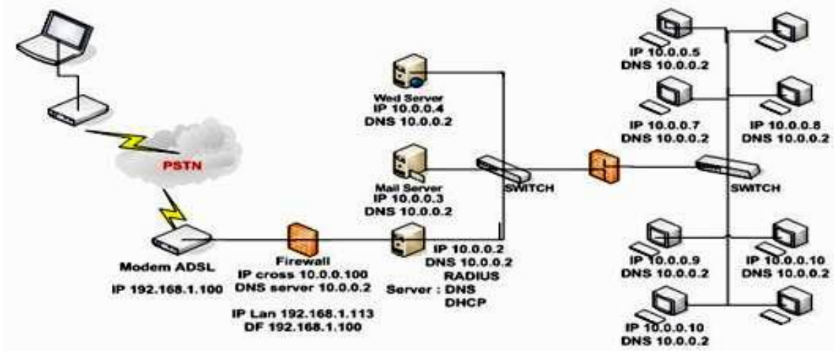
Hình 6.6 - Mô hình Firewall phức tạp thường sử dụng trong các doanh nghiệp lớn
