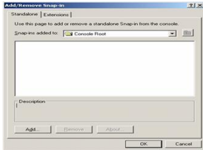
Hình 8.32 - Add Snap-in
