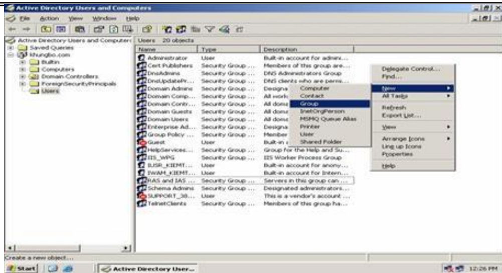
Hình 8.2 – Tạo Group
