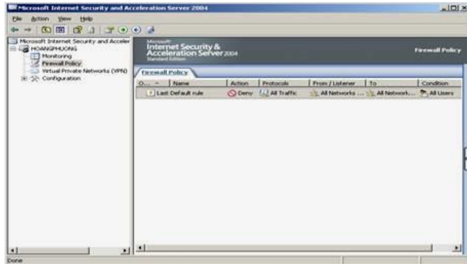
Hình 7.6 – Rule mặc định trong Firewall Policy
