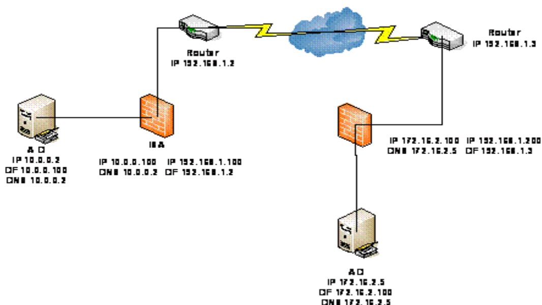
Hình 8.50 - Mô hình VPN Site to Site
