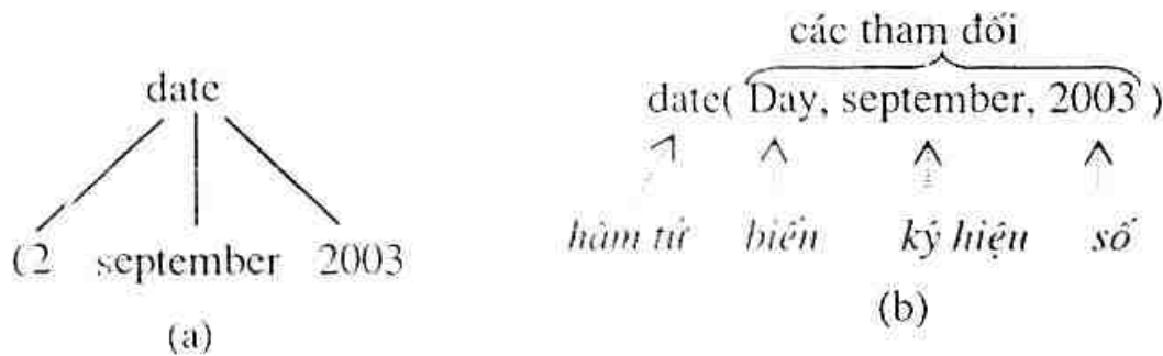
Hình 1.9. Ngày tháng là một đối tượng có cấu trúc:
