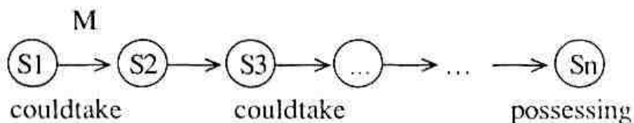
Hình 2.10. Dạng đệ quy của vị từ couldtake
