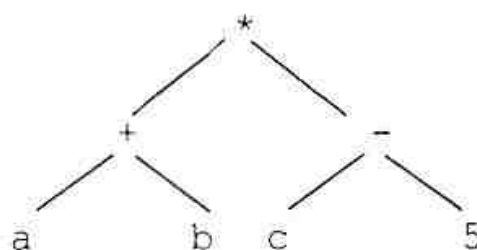
Hình 1.12. Cấu trúc cây của biểu thức (a + b) * (c - 5)
