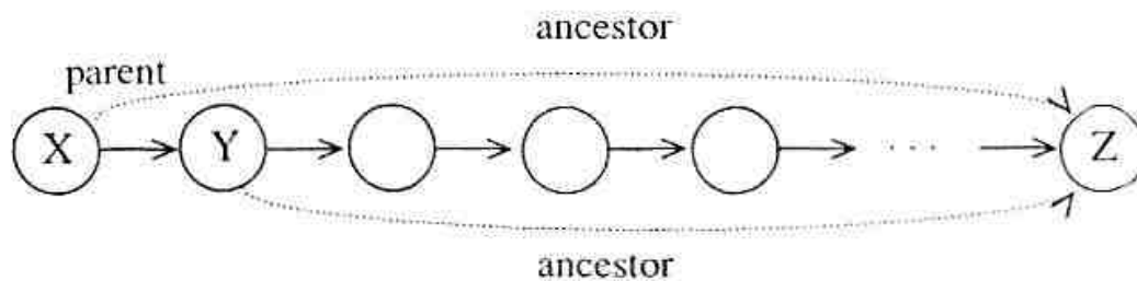
Hình 1.8. Dạng đệ quy của quan hệ tổ tiên (được quay ngang cho thuận tiện)
