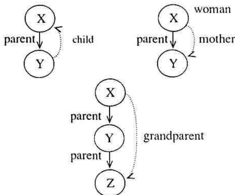
Hình 1.4. Định nghĩa quan hệ con, mẹ và ông bà sử dụng một quan hệ khác
