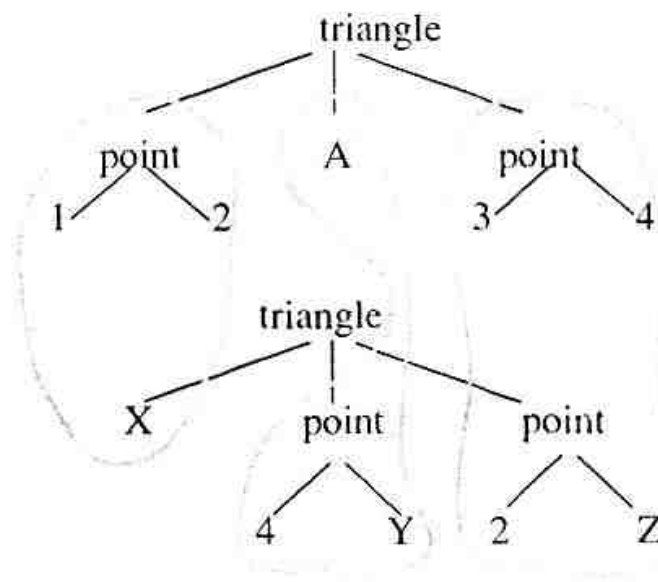
Hình 1.13. Kết quả so khớp:
