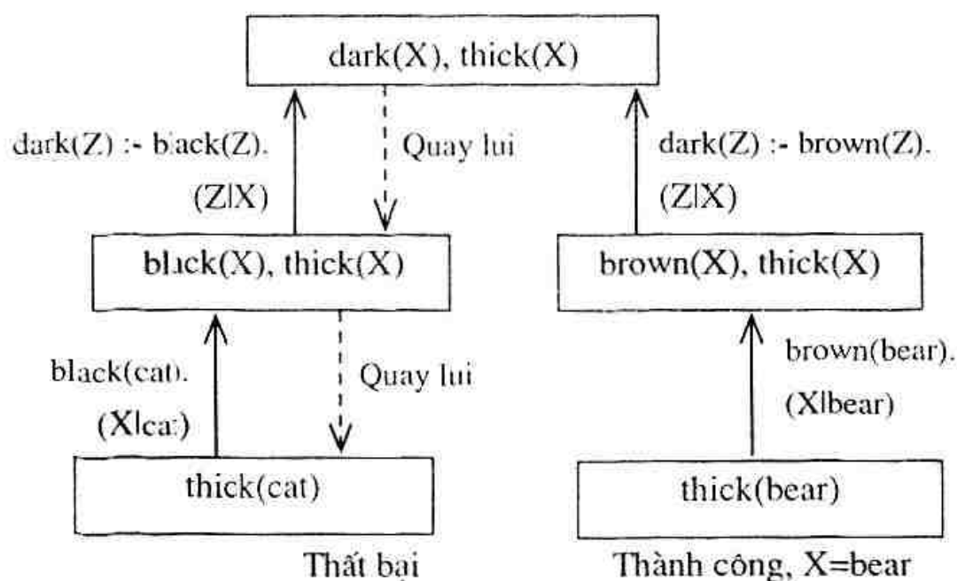
Hình 2.6. Quá trình thực hiện xoá đích dark(X), thick(X)
