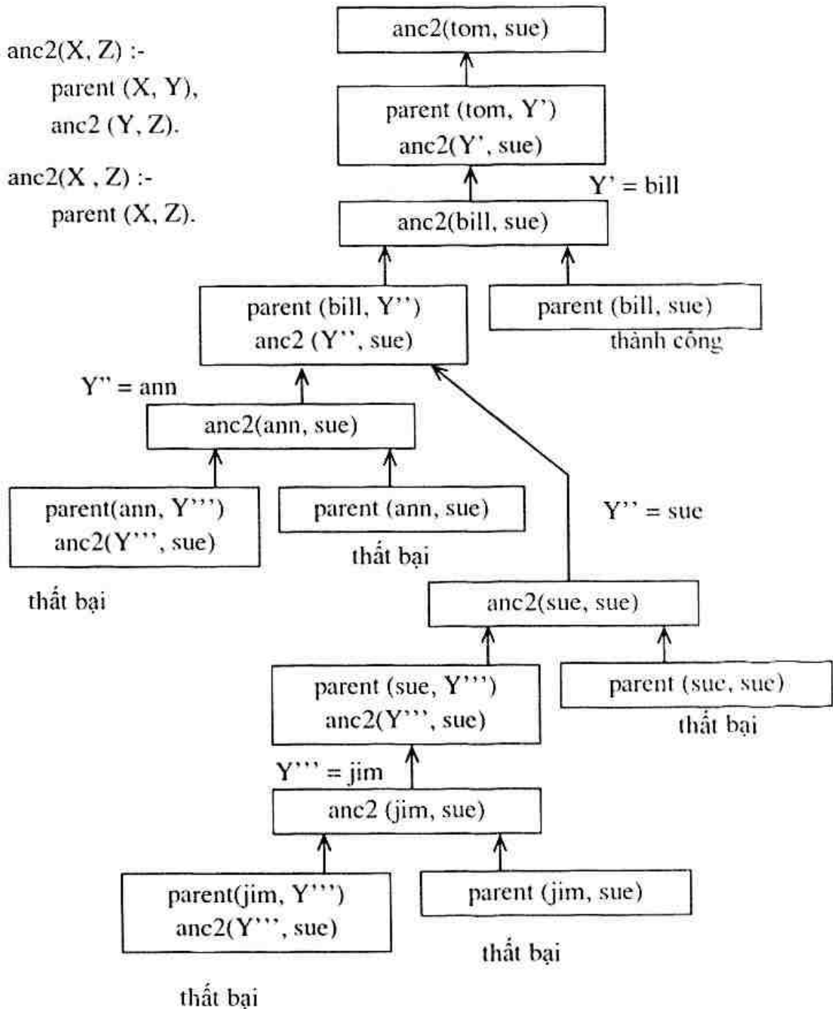
Hình 2.12. Biểu thể a của quan hệ tổ tiên trả lời câu hỏi "Tom có phải là một tổ tiên của Sue ?"
