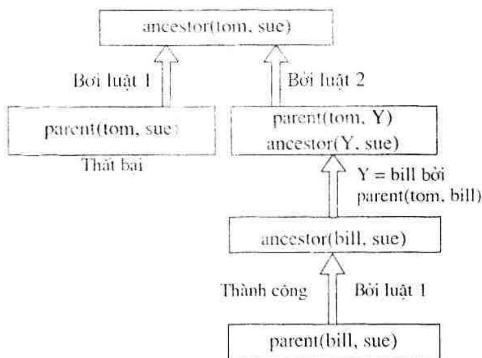
Hình 2.4. Quá trình thực hiện xóa đích ancestor(tom, sue)
