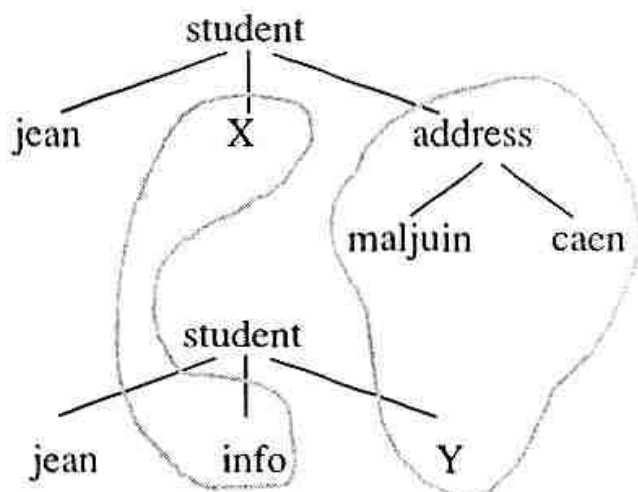
Hình 1.15. Kết quả so khớp:
