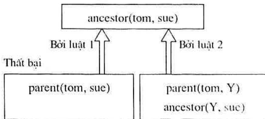
Hình 2.3. Các giai đoạn thực hiện xử lý xoá đích
