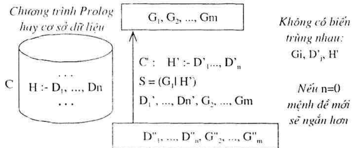
Hình 2.5. Quá trình thực hiện execute
