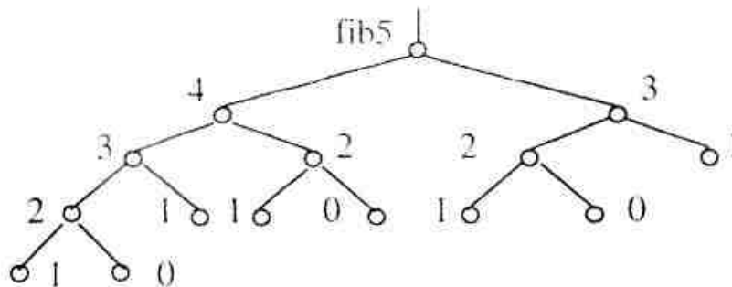
Hình 3.5. Biểu diễn cây các lời gọi đệ quy tìm số Fibonacci
