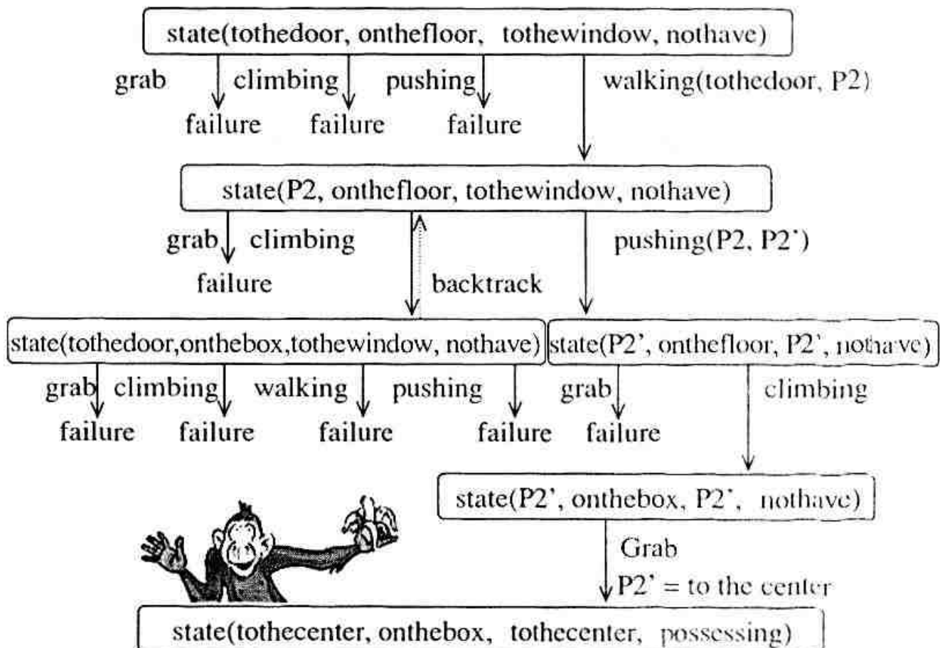
Hình 2.11. Lời giải của bài toán con khỉ và quả chuối.
