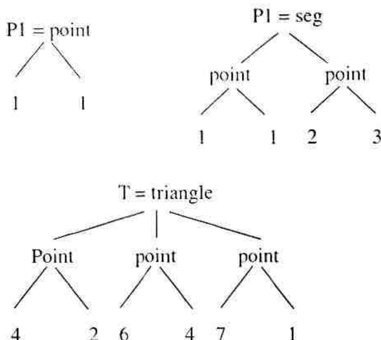
Hình 1.11. Biểu diễn dạng cây của các đối tượng
