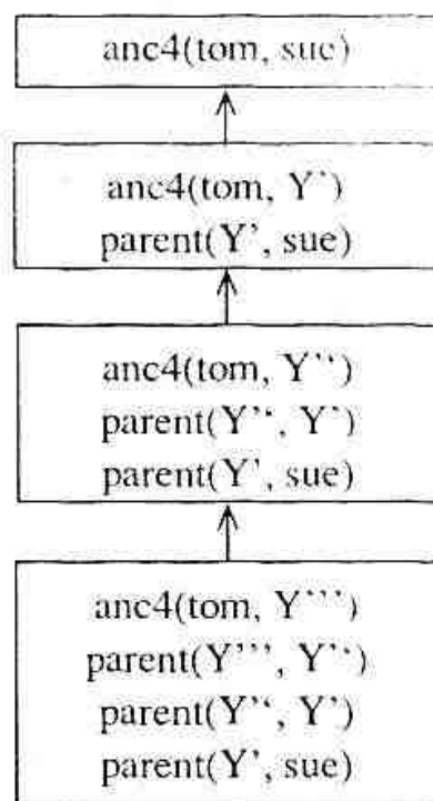
Hình 2.14. Biểu thể c của quan hệ tổ tiên trả lời câu hỏi "Tom có phải là một tổ tiên của Sue ?"
