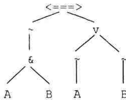
Hình 3.4. Biểu diễn cây của hạng \sim (A \& B) \<==> \sim A \vee \sim B
