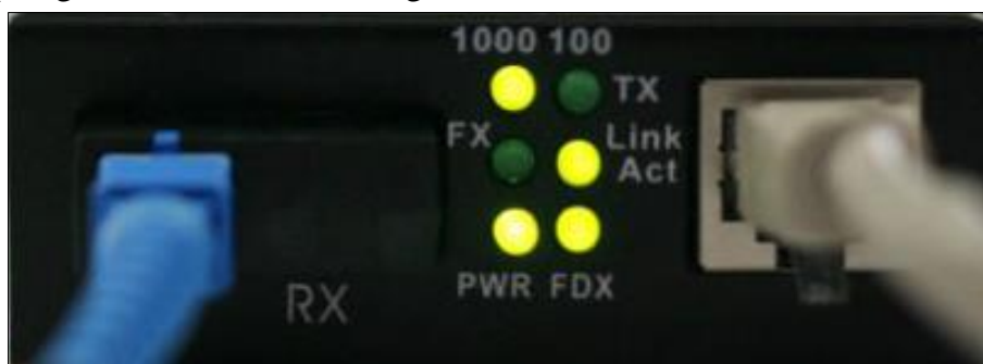
Hình 4.6 Converter quang – Bộ chuyển đổi quang điện 1G khi mất tín hiệu quang Khi mất kết nối LAN từ Switch đến Converter quang điện 2 đèn hàng TX sẽ tắt, lúc này chỉ còn FX và đèn nguồn trên Converter quang sáng
