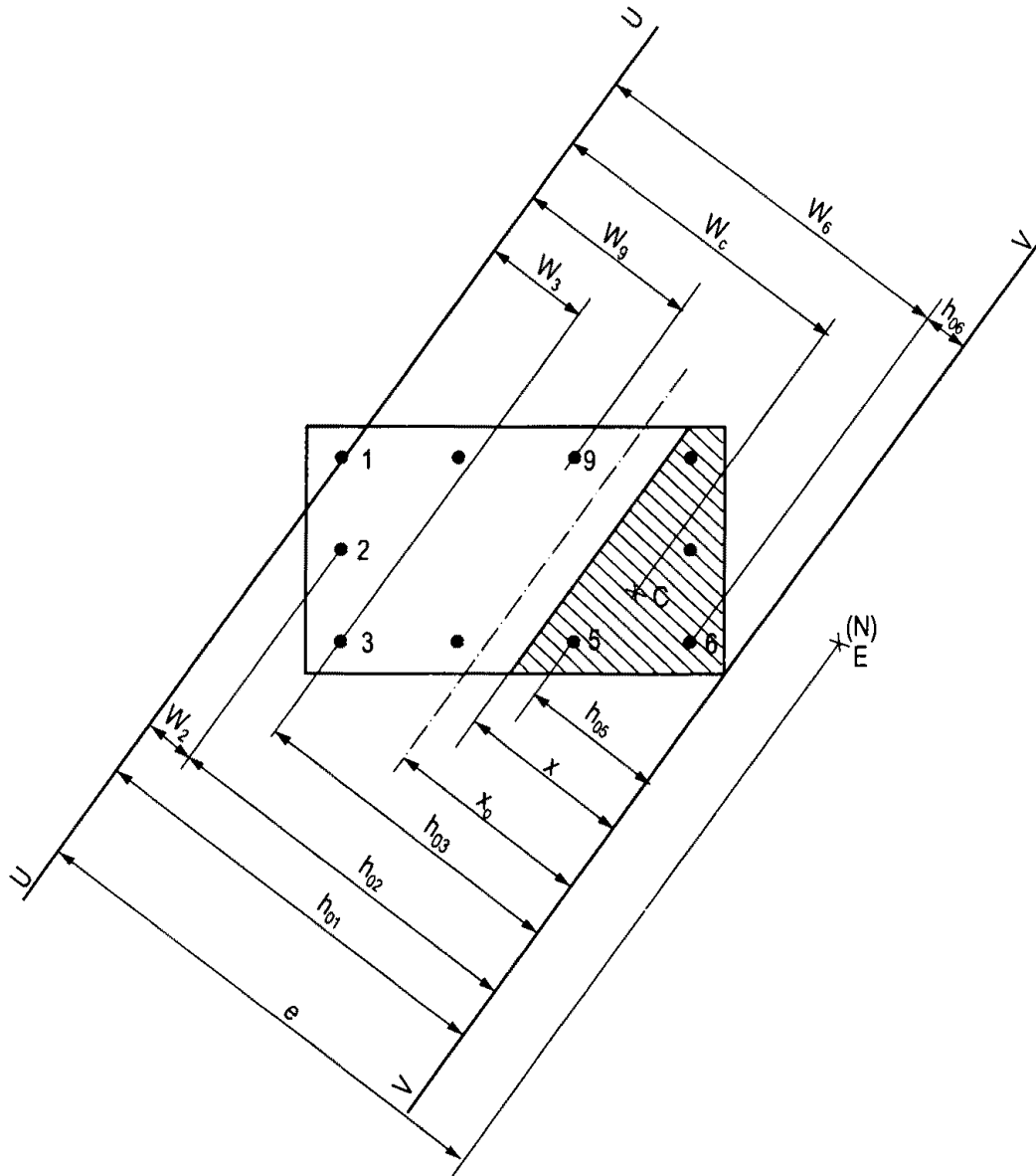
Hình 5.5. Sơ đồ tính toán của tiết diện
