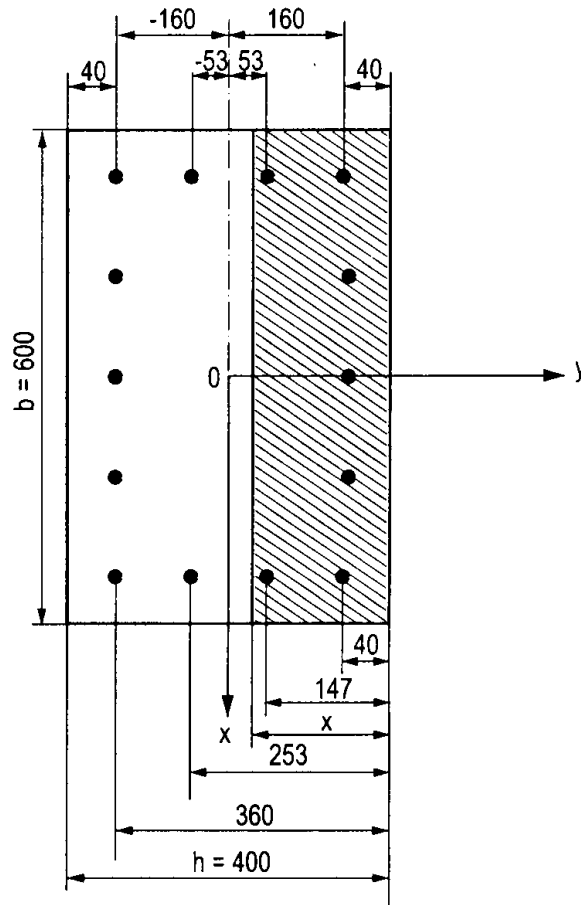
Hình 5.17. Sơ đồ tính N_y
