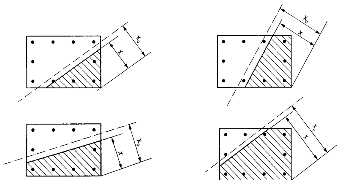
Hình 5.4. Các dạng của vùng nén
