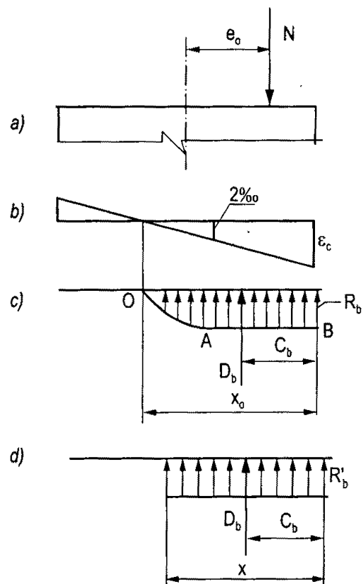
Hình 1.24. Ứng suất trong bê tông vùng nén: a) Sơ đồ nội lực; b) Biểu đồ biến dạng; c) Biểu đồ ứng suất thực; d) Biểu đồ đơn giản hóa.
