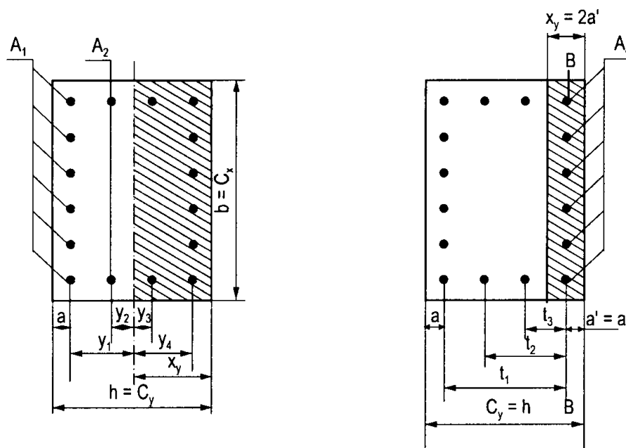
Hình 5.15. Sơ đồ tính M_{By} , M_{Dy}
