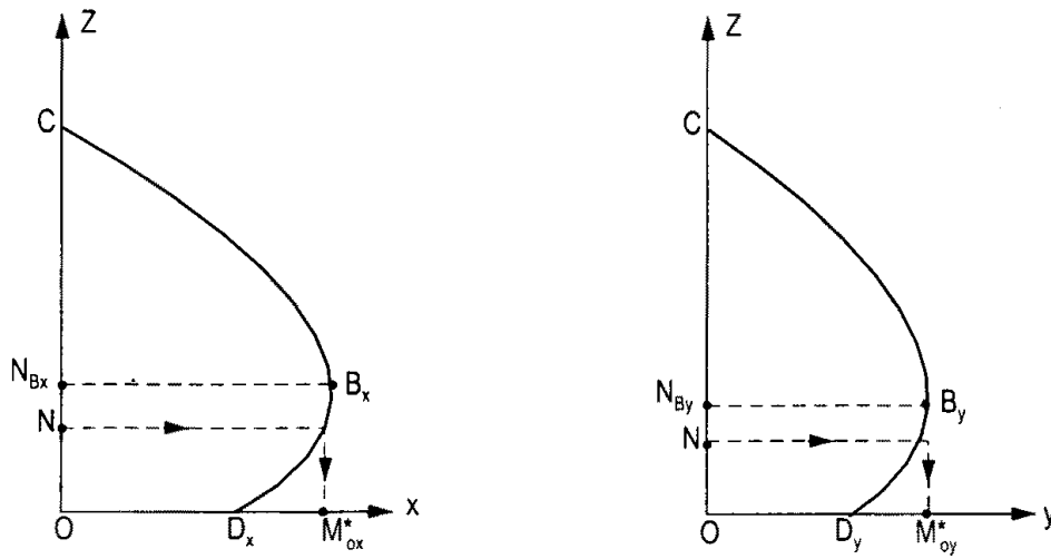
Hình 5.13. Sơ đồ xác định M_{ox}^* và M_{oy}^*
