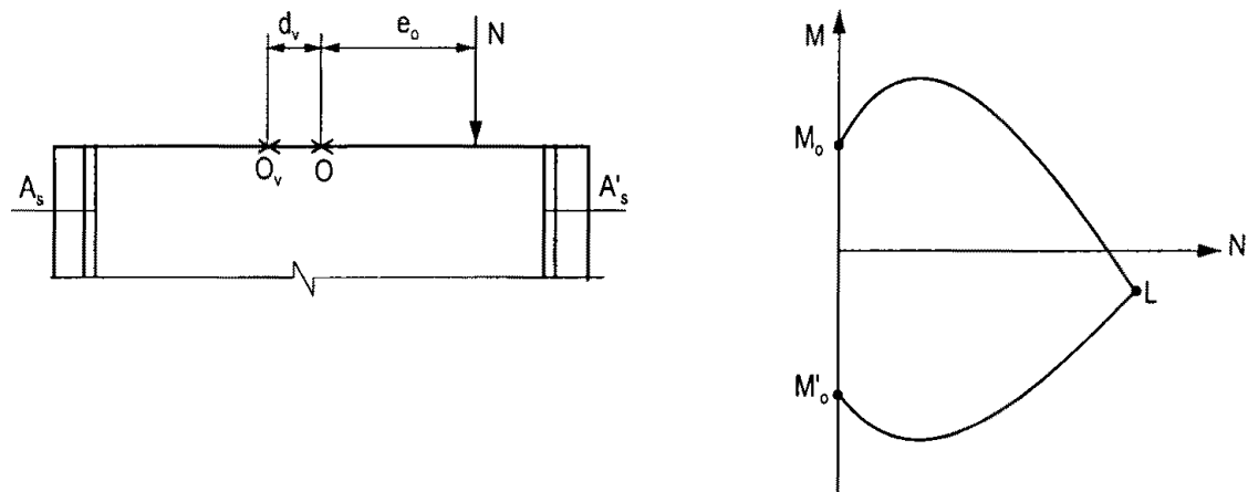
Hình 2.12. Sơ đồ và biểu đồ tương tác khi A_s > A'_s
