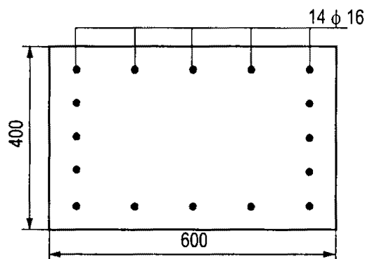
Hình 5.11. Tiết diện cột của thí dụ 2
