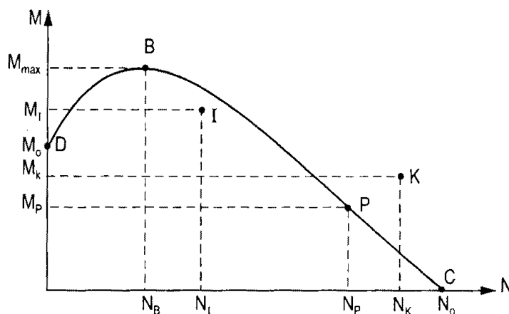
Hình 2.9. Biểu đồ và các cặp nội lực
