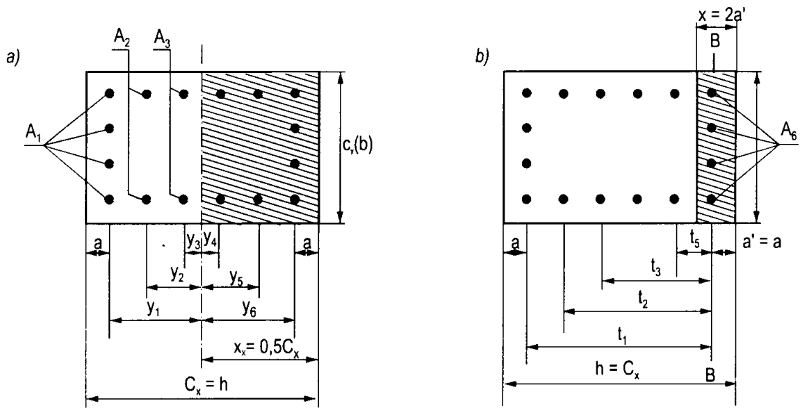
Hình 5.14. Sơ đồ tính M_{Bx} và M_{Dx}
