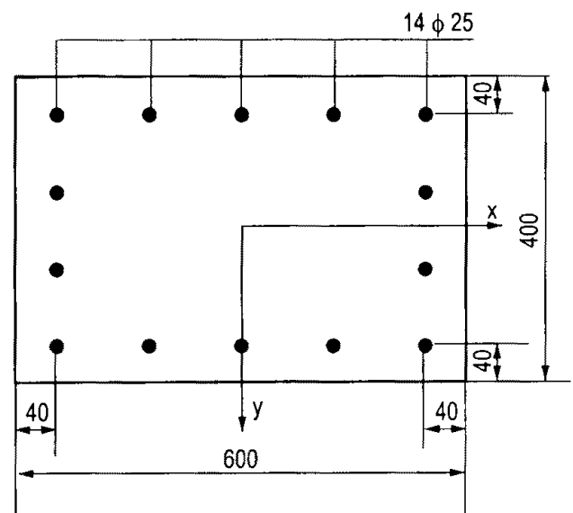
Hình 5.16. Hình vẽ của thí dụ 1
