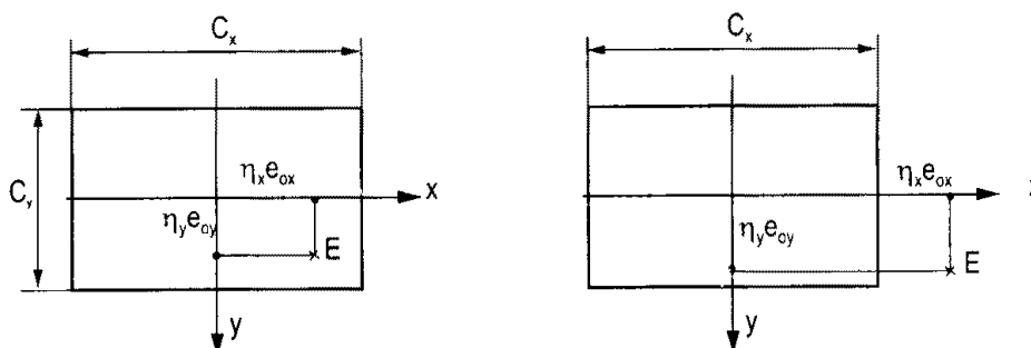
Hình 5.3. Sơ đồ nội lực với độ lệch tâm
