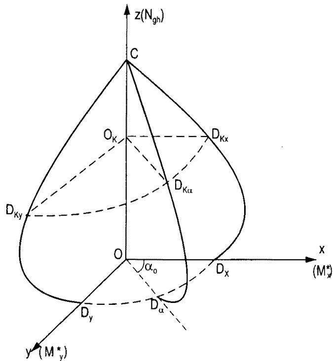
Hình 5.7. Mặt biểu đồ tương tác
