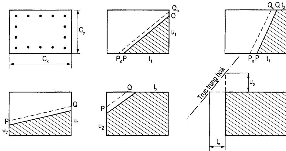
Hình 5.8. Dạng và kích thước vùng nén
